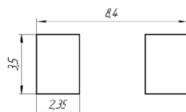
РАСПОЛОЖЕНИЕ КОНТАКТНЫХ ПЛОЩАДОК
